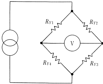
(b) Y軸検出回路
