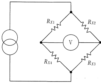
(a) X軸検出回路
