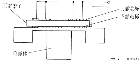
図1 断面図
