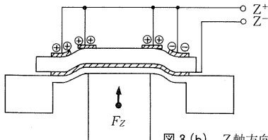
図3(b) Z軸方向加速度
