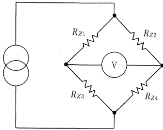
(c) Z軸検出回路
